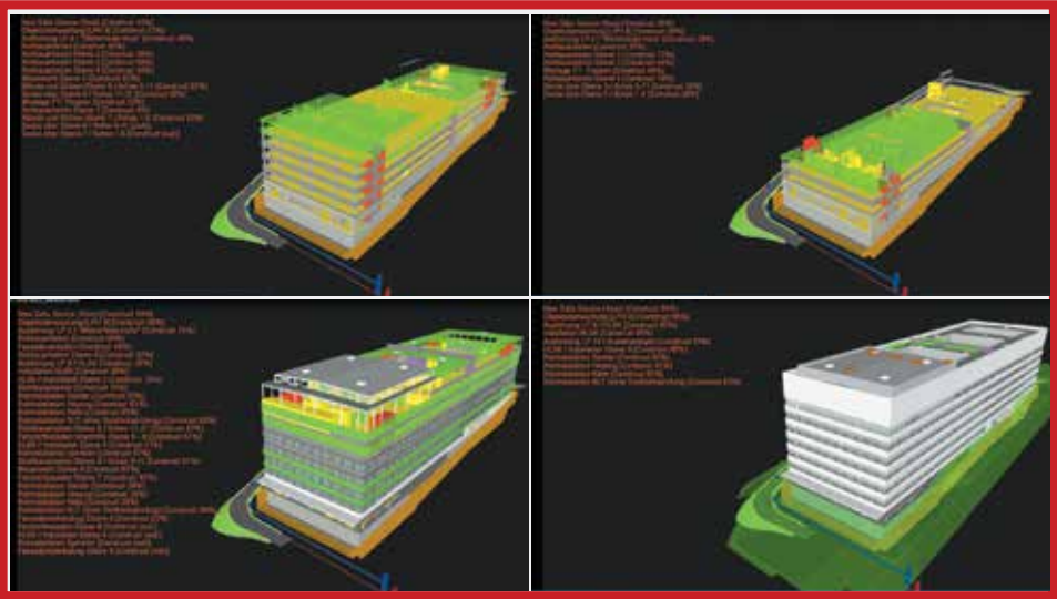
BIM Modell eines Bauprojektes der Bayer AG in Wuppertal Quelle: Bayer AG / C&P / formitas
